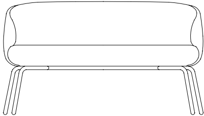
GZ6400 W 52 D 23 H 30 SH 19.25
